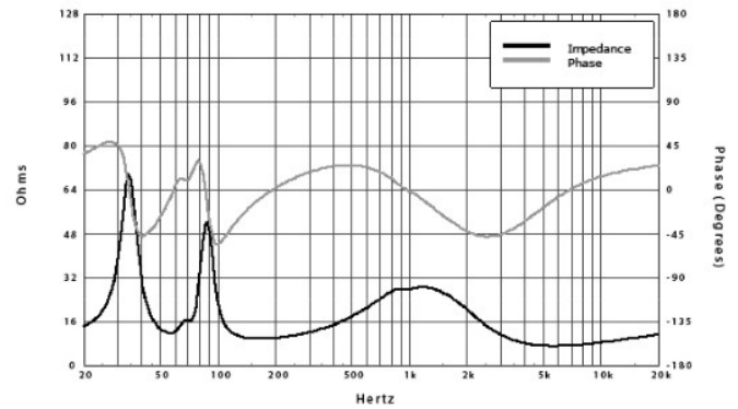
Impedance/Phase
